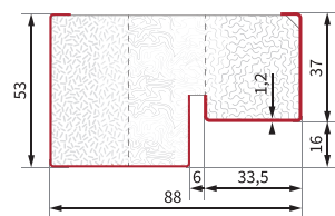
Przekrój profilu ościeznicy drewniano-stalowej TERMA .
