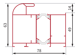
Przekrój profilu ościeznicy aluminiowej.
