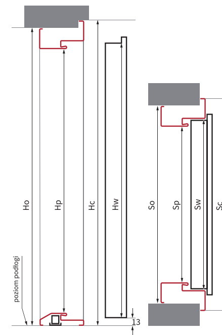
Schemat ościeżnicy C (przekrój pionowy i poprzeczny).
