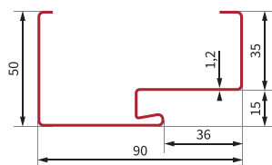
Przekrój profilu ościeznicy stalowej B .
