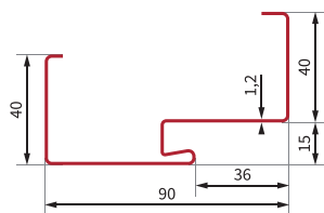
Przekrój profilu ościeznicy stalowej C (standard).
