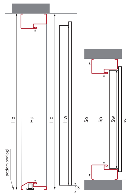
Schemat ościeżnicy B (przekrój pionowy i poprzeczny).
