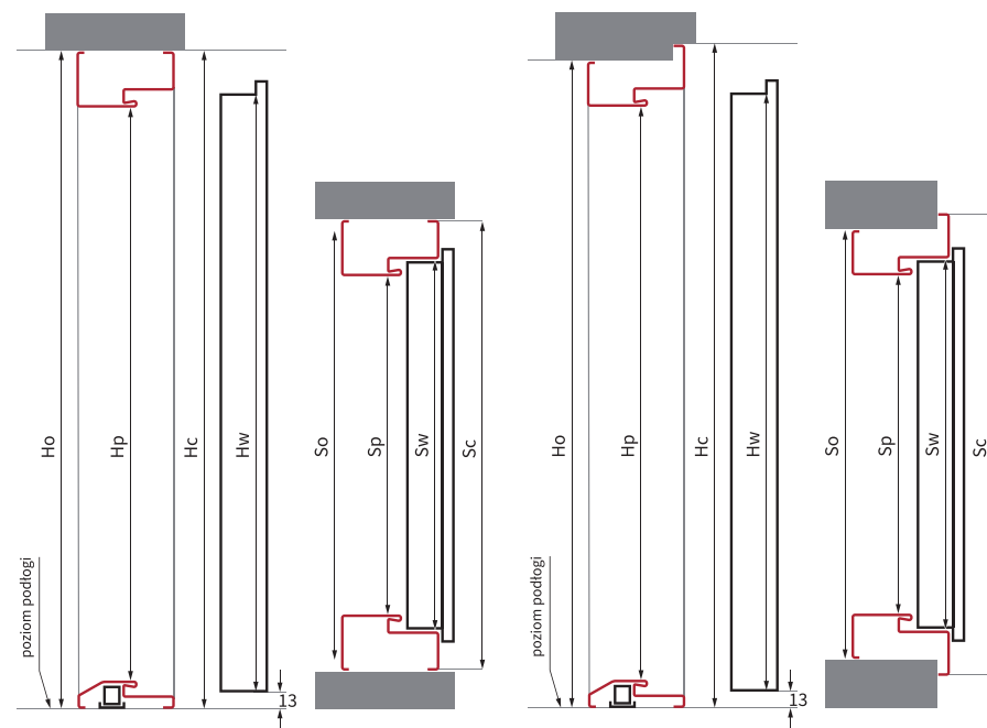
Schemat ościeżnicy B i TERMA (przekrój pionowy i poprzeczny). Schemat ościeżnicy C (przekrój pionowy i poprzeczny).
